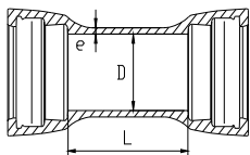
K=12
